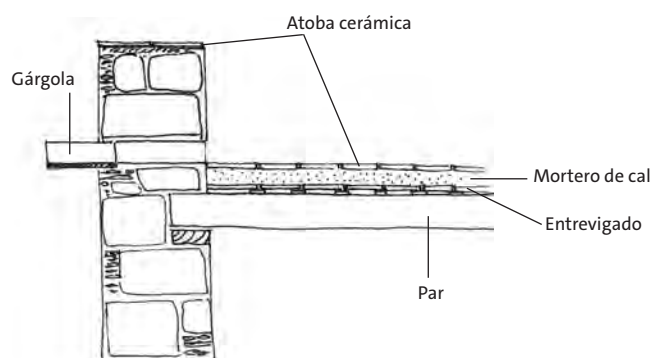
Detalle tipo de cubierta plana con acabado de atoba cerámica.
