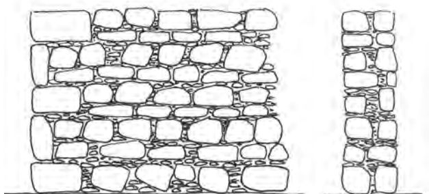
Sección y alzado de mampostería tipo A-1 por hiladas horizontales. Elaboración propia
