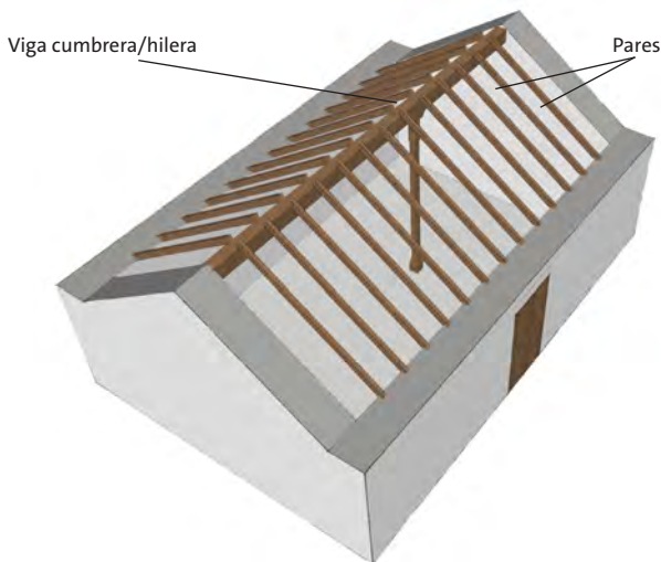
Esquema de cubierta par e hilera.
