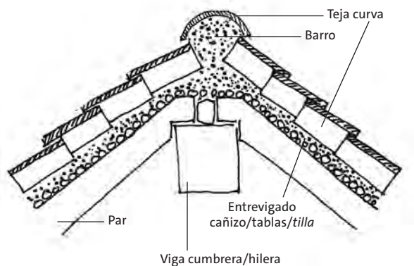
Sección detalle de cumbre.
