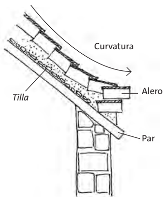
Detalle de encuentro de estructura de cubierta con muro lateral: par que sobresale del muro.
