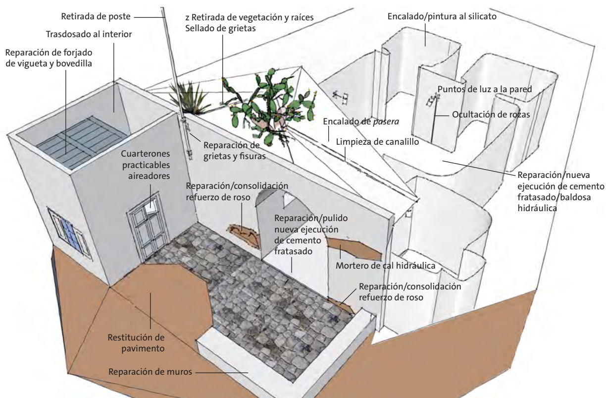
Materiales y técnicas de rehabilitación de casa-cueva.
