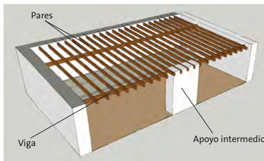
Esquema de cubierta a un agua par sobre viga doble con apoyo intermedio.
