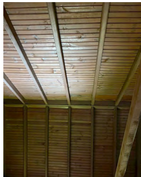
Entrevigado con paneles prefabricados de madera en cubierta de par e hilera con solera y tirante. Vigas tratadas con lasur coloreado.
