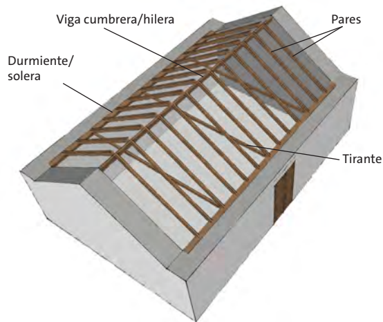
Esquema de cubierta a dos aguas, par e hilera con durmiente y tirante.
