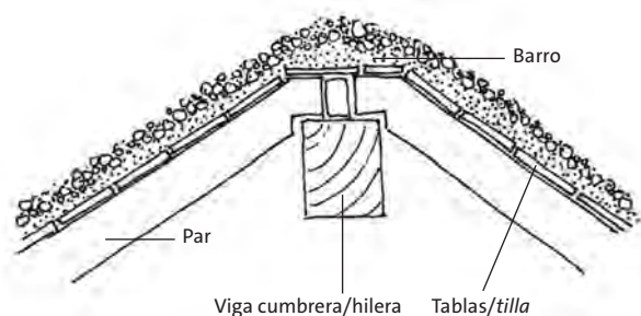
Detalle de cumbrera de cubierta de tierra.
