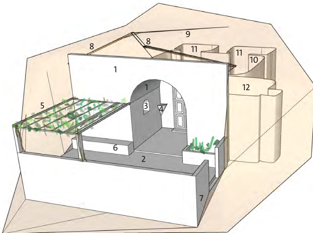
Casa-cueva esquema b: 1. Roso, 2. Patio, 3. Alacena para bernegal/talla, 4. Repisa, 5. Latada , 6. Banco, 7. Zona de relleno, 8. Canales de drenaje, 9. Pasera , 10. Estancia principal (interior), 11. Aposento (interior), 12. Cocina (interior).
