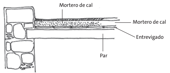
Detalle tipo de cubierta plana con acabado mortero de cal/tierra.
