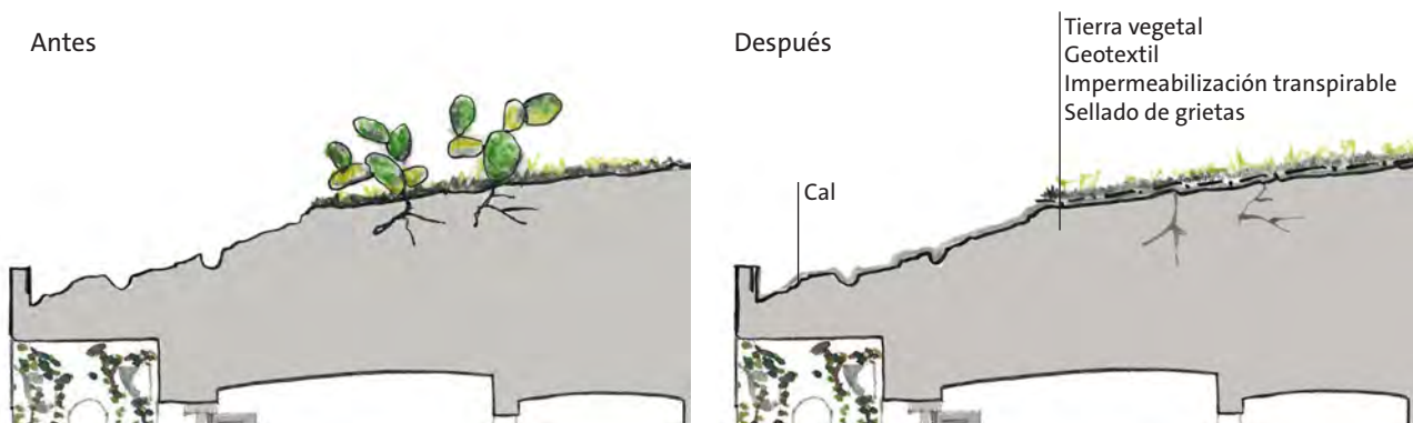
Antes y después de intervención en techo y pasera
