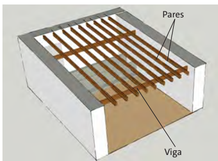
Esquema de cubierta a un agua par sobre viga sencillo.
