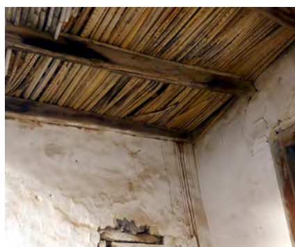
Reposición de entrevigado con pírgano , El Parralillo, Santa Lucía.
