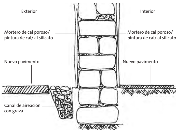
Detalle de posibles soluciones a la humedad por capilaridad en muros.
