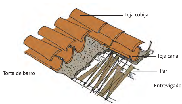
Sección del tejado con teja curva.
