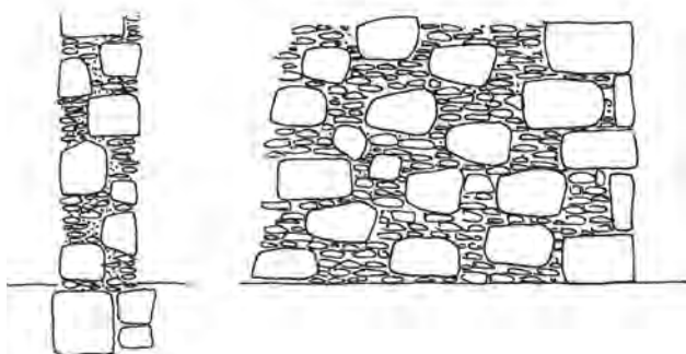
Sección y alzado de mampostería tipo A. Elaboración propia.
