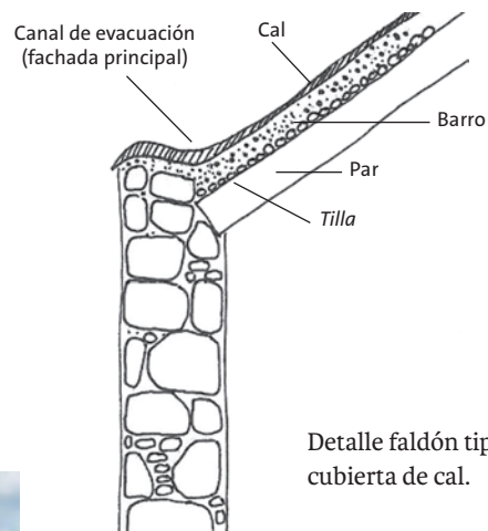
Detalle de evacuación de aguas del faldón en cubierta a dos aguas de cal.
