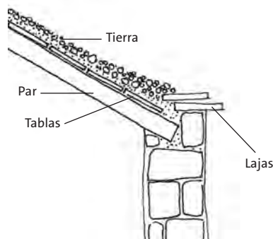
Detalle faldón tipo cubierta de tierra.
