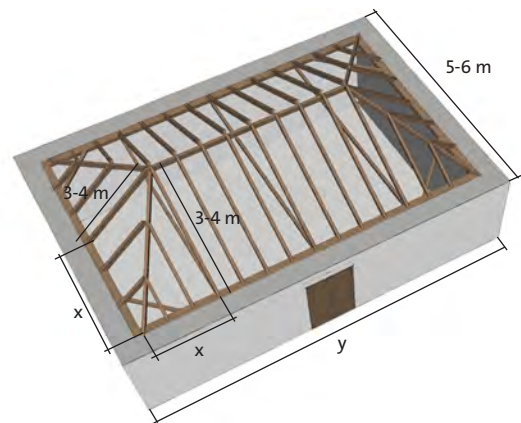
Esquema de cubierta a cuatro aguas, par e hilera con durmiente, tirante y cuadrante.
