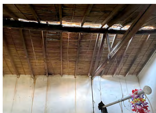
Entrevigado de cañizo con atado intermedio, Ventanieves, Vega de Acusa.
