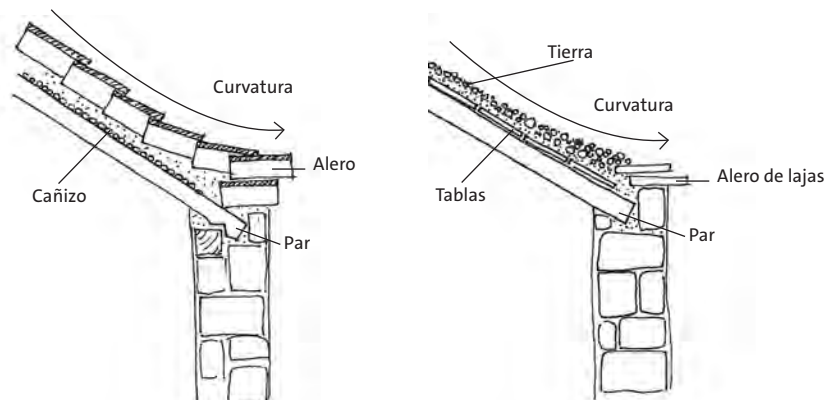
Detalle de encuentro de estructura de cubierta con muro lateral: par embebido en el muro. A: par sobre durmiente, cañizo, torta de barro y tejas. B: par e hilera, tablas y tierra con alero de lajas.
