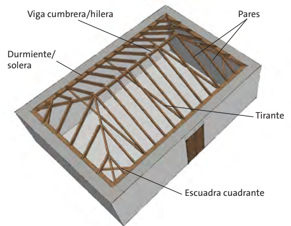
Esquema de cubierta a cuatro aguas, par e hilera con durmiente, tirante y cuadrante.
