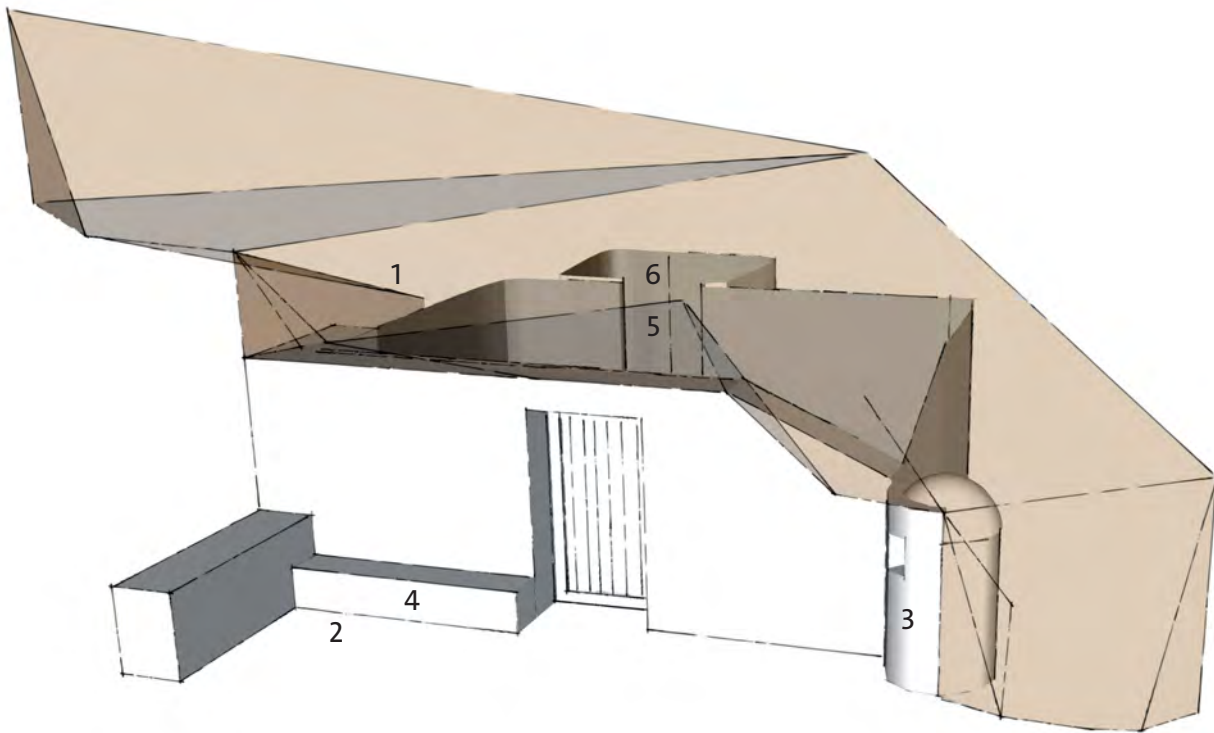
Casa-cueva esquema a: 1. Roso, 2. Patio, 3. Horno, 4. Banco, 5. Habitación principal (interior), 6. Aposento (interior).
