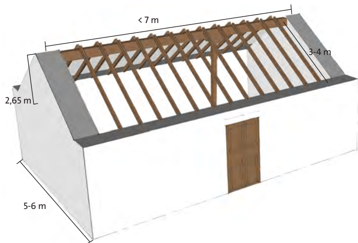
Apeo con pie derecho a un tercio, Hoya Grande, Tunte.
