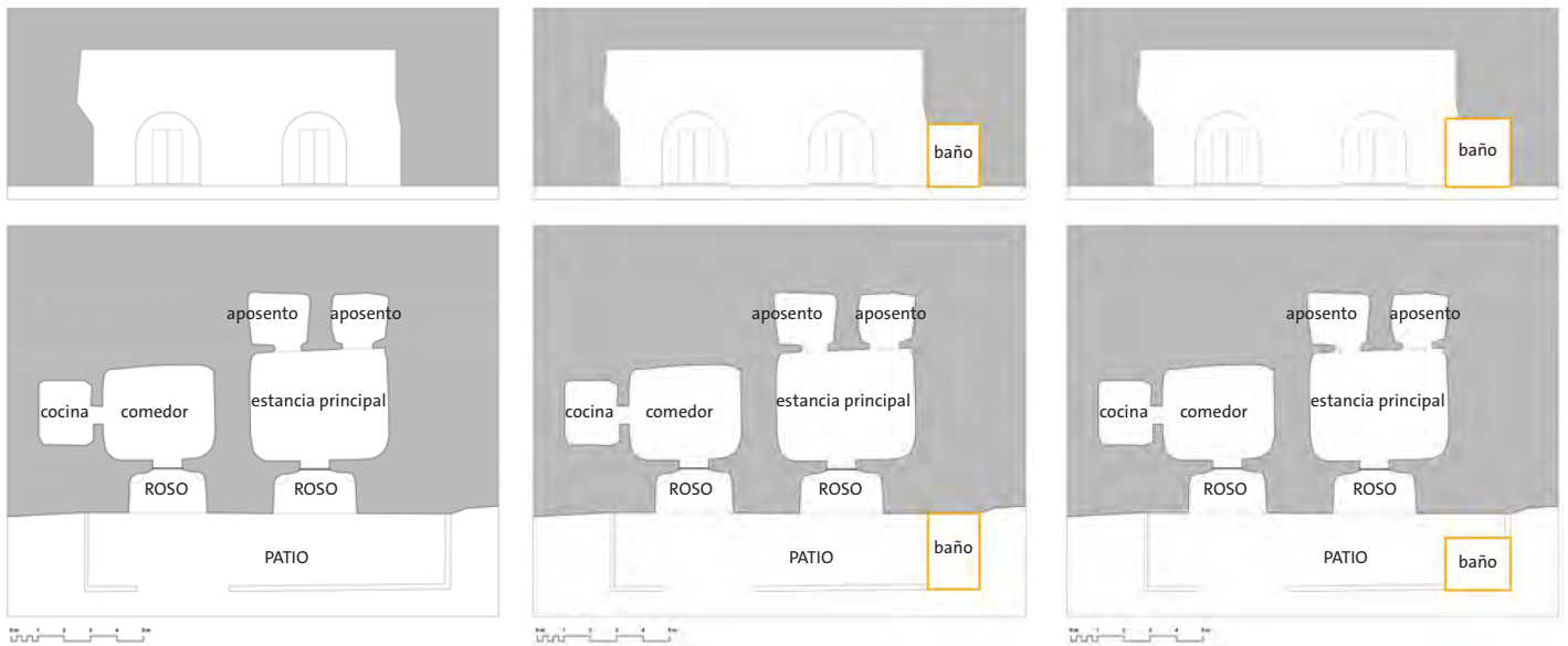
Esquema de casa-cueva de roso de mampostería abovedado: estado actual-propuestas A (baño adosado fuera del frontis) y B (baño exento).
