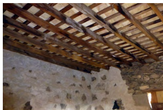
Entrevigado de atoba cerámica, Los Rosales, Fingas.
