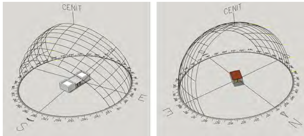
Orientación y soleamiento de alpende en El Lirón, Ingenio, sol en cenit, 21 de junio y alpende en Trasmontaña, Arucas, sol en cenit, 21 de diciembre.
