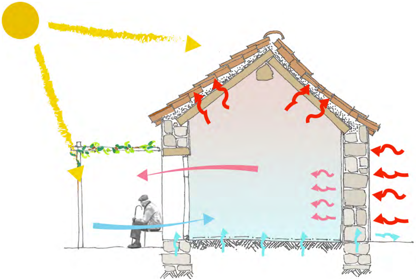
Esquema bioclimático de la vivienda rural.
