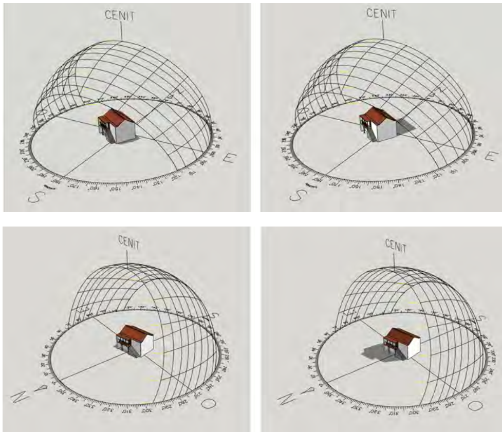
Orientación y soleamiento de vivienda con galería en Arucas (UTM: 447738.80, 3110999.71, altitud: 193m), sol en cenit, 21 de junio y 21 de diciembre.
