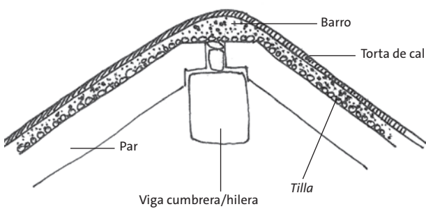
Detalle de cumbre de cubierta de cal.
